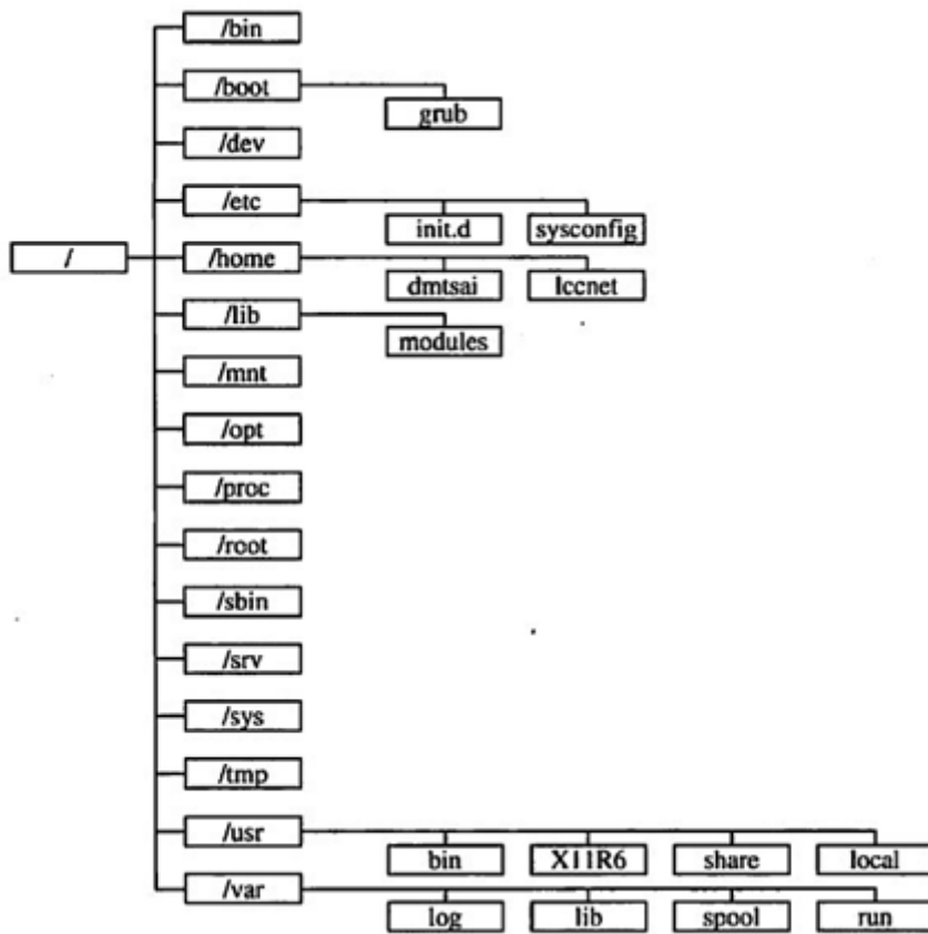
图 6-1 Linux 系统目录结构图
