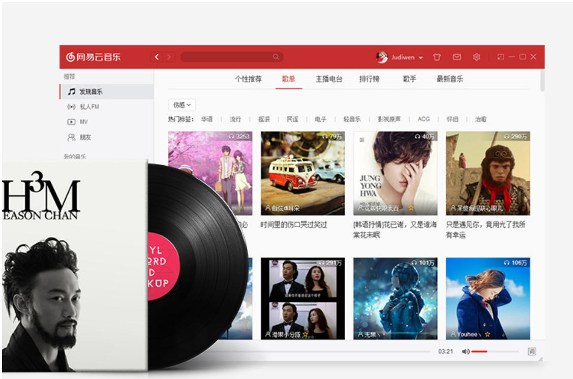
图 3-13 网易云音乐
