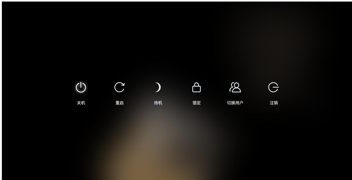
图 3-8 关机
