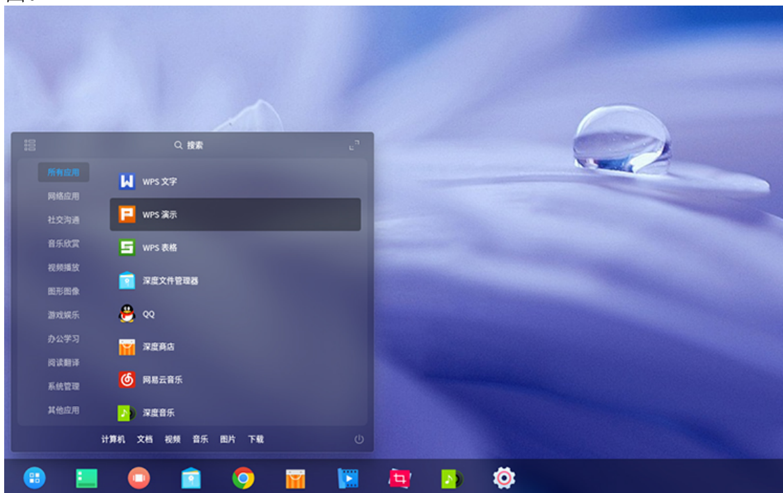
图 3-6 启动项
