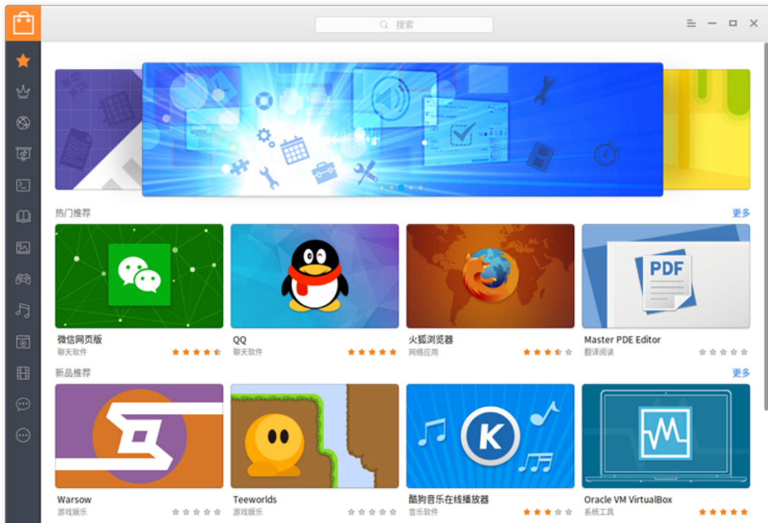
图 3-11 深度商店
