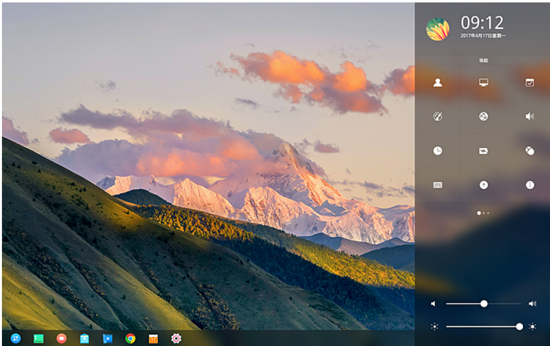
图 3-9 控制中心
