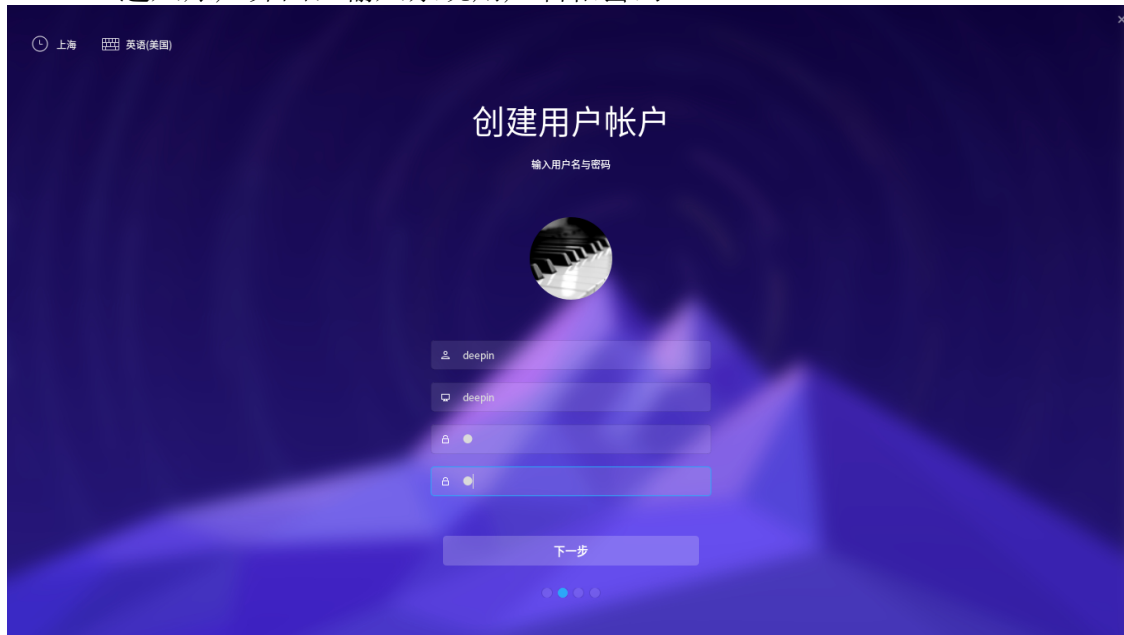
图 3-4 账户界面
