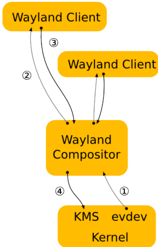
图 2-3 Wayland 架构图
