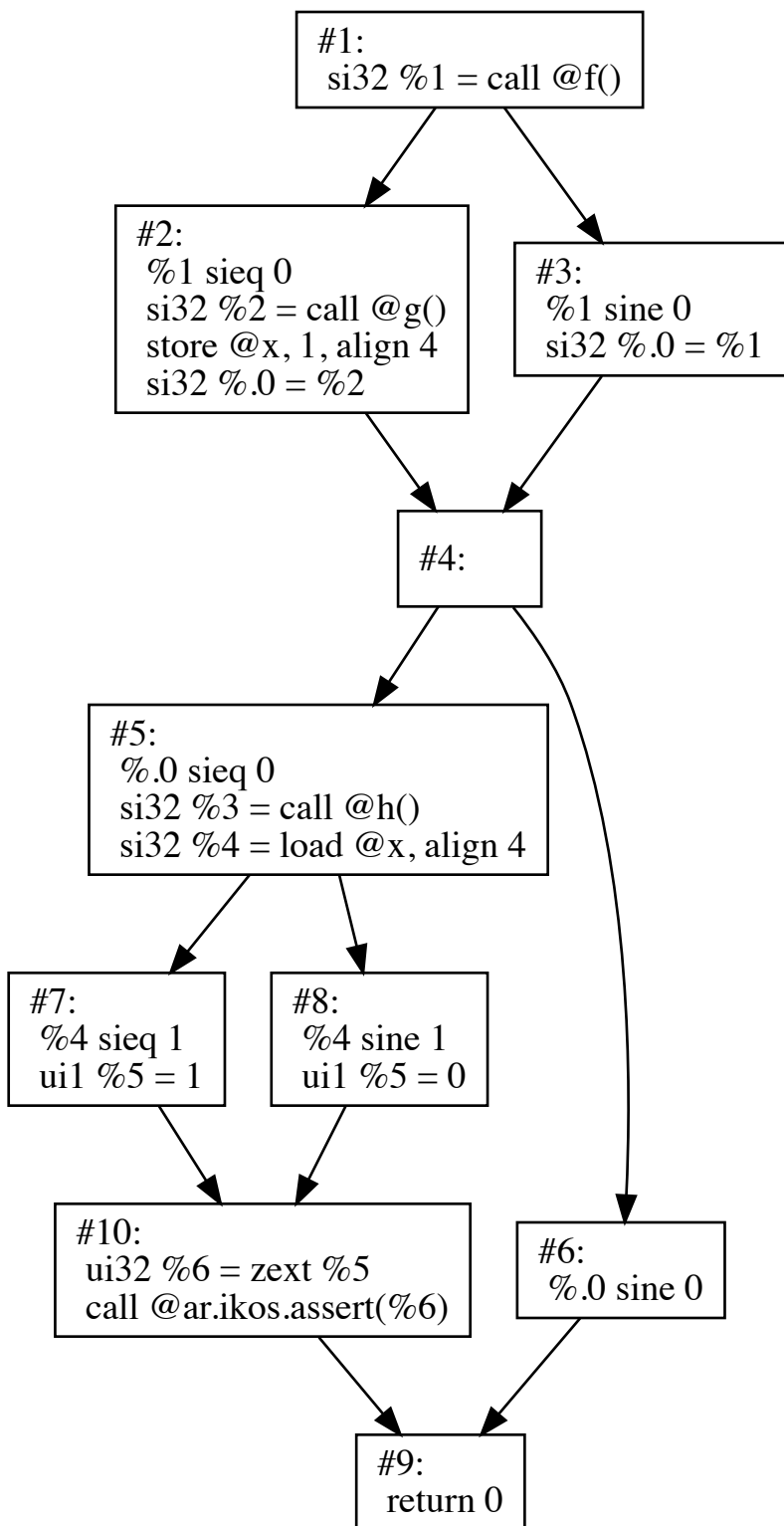
CFG for 'main' function
