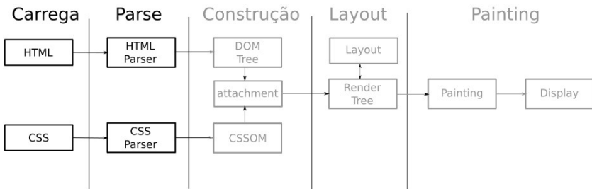
Figura 9.5: Parse dos dados
