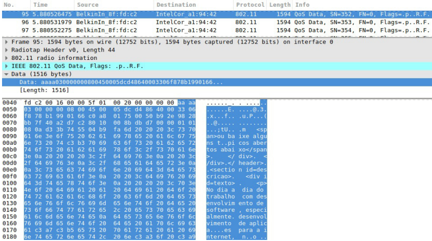
Figura 6.13: Dados dentro de uma conexão WPA2 com HTTP quando temos a senha
