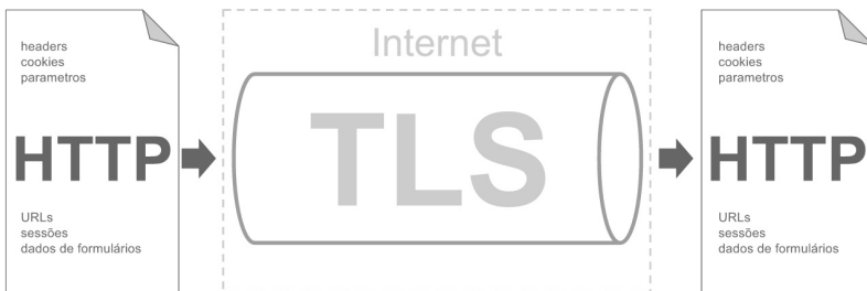
Figura 5.17: Informações protegidas
