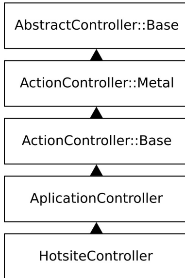
Figura 8.7: Herança do controller do desconstruindoaweb no Rails
