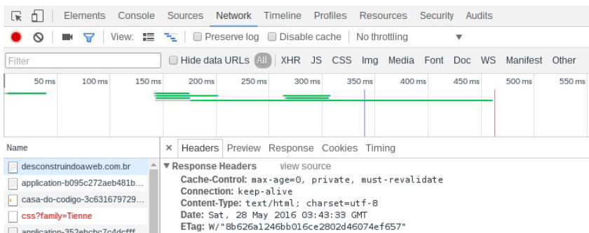
Figura 1.9: Cabeçalhos de cache no developer tools do Chromium em uma requisição real
