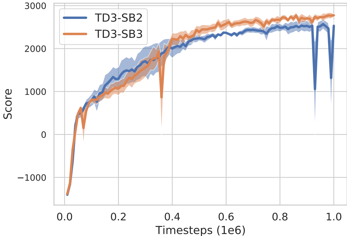
HalfCheetahBulletEnv-v0
